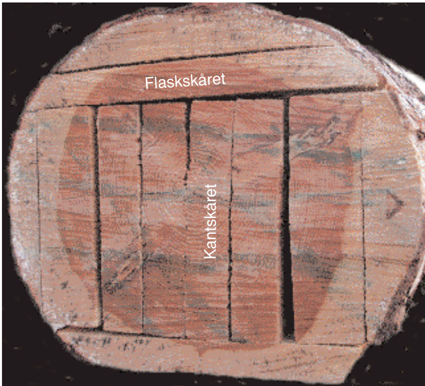
Bildet viser tverrsnittet av en stokk og hvordan en kan legge opp skuren på saga for å få høy andel av kantskårne bord og mye kledning av kjerneved. Her er det skåret 25 mm x 150 mm kledning ut av sentrumsuttaket. Det bør være 20 cm kjerneved for å klare dette.
